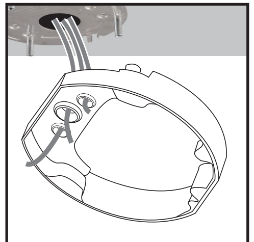
ケーブルを通すイメージ図
